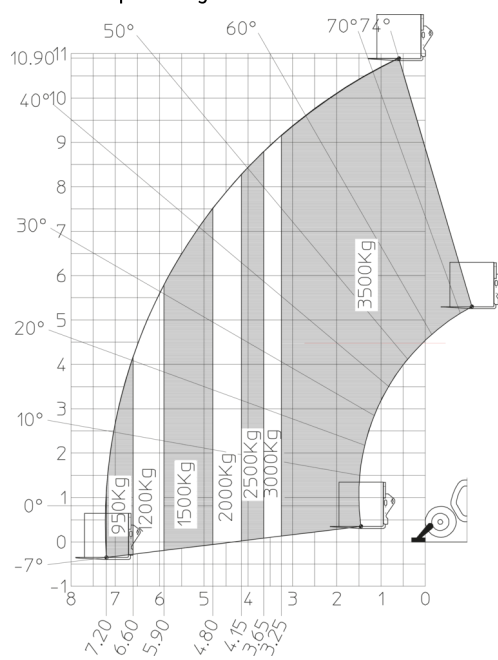
Rotatie op verlaagde stabilisatoren met vorken
