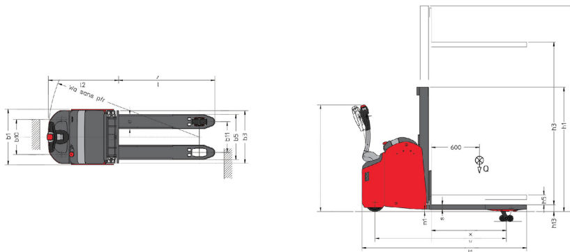
ES 420 DL PFR 6 - Tekening met afmetingen
